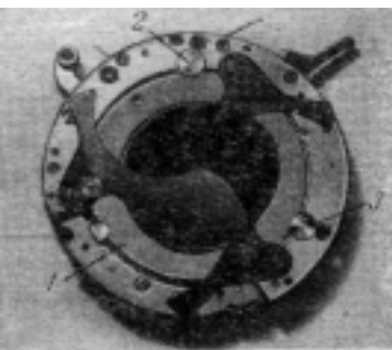
Рис. 48. Лепестки затвора
