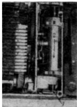
Рис. 128. Смещение зубчатого валика по стрелке
