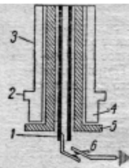
Рис. 50. Схема синхроконтактного гнезда
