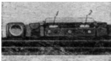
Рис. 40. Опорные точки прицельной рамки
